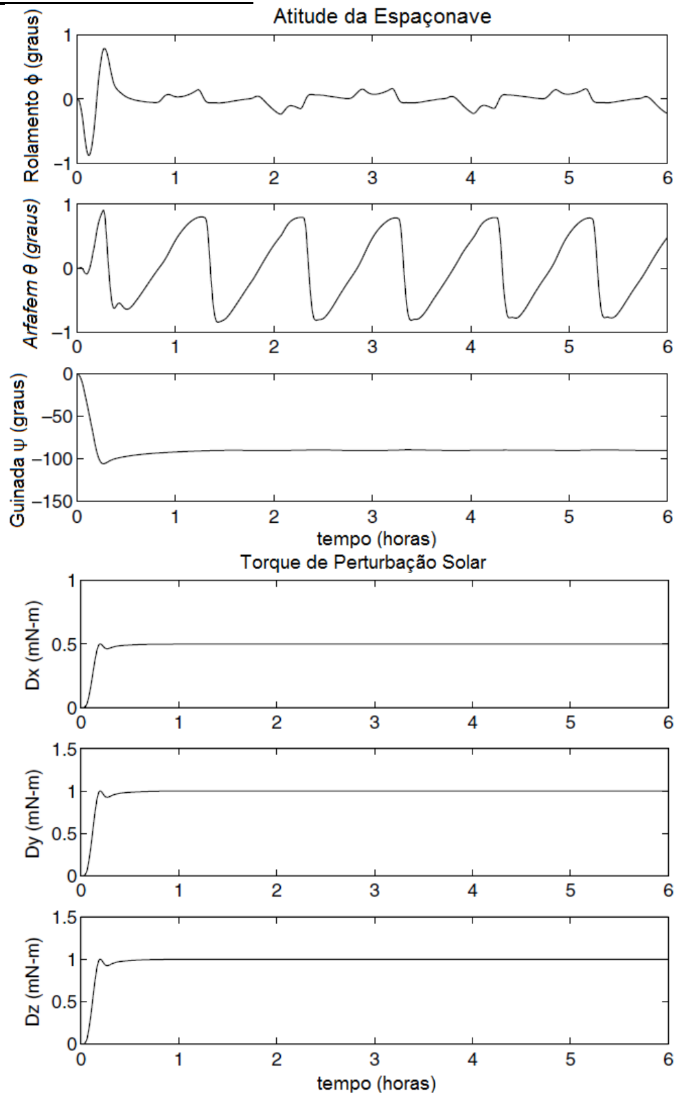
Figura 1. Uma manobra de 90° de guinada de uma vela solar de 40 m (com \epsilon = 0,1 m), utilizando RRs e TMs para uma transição do modo de empuxo zero para o modo de espera empuxo total. [Fonte: Wie, 2008]
